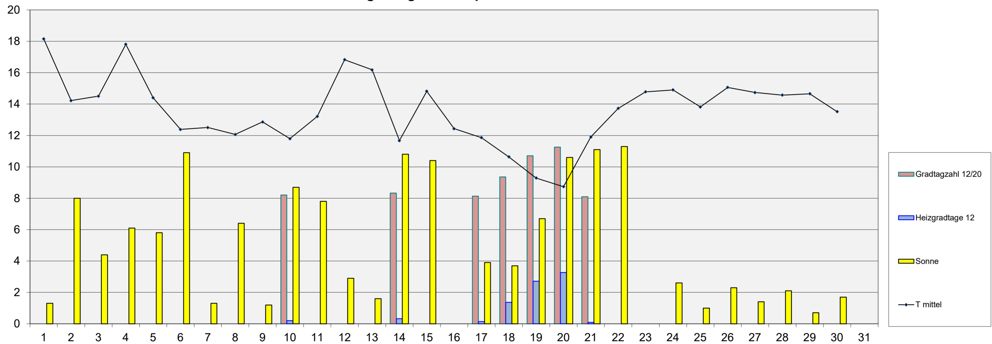
Energiediagramm September 2019
