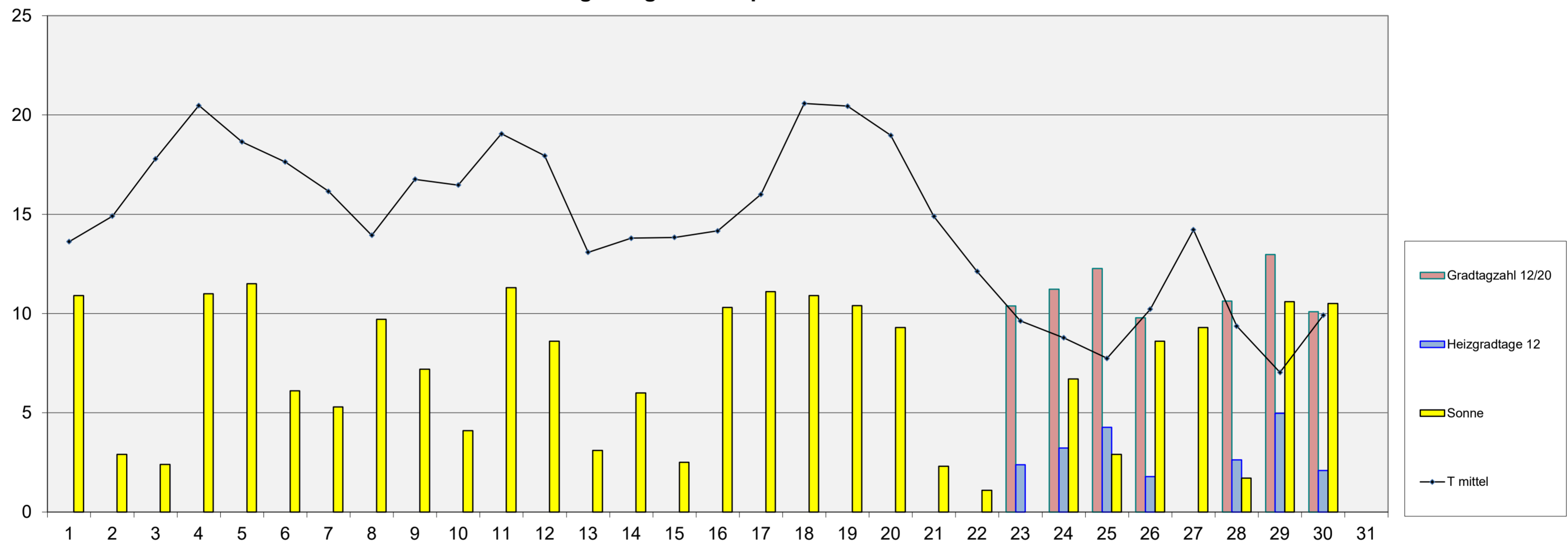
Energiediagramm September 2018
