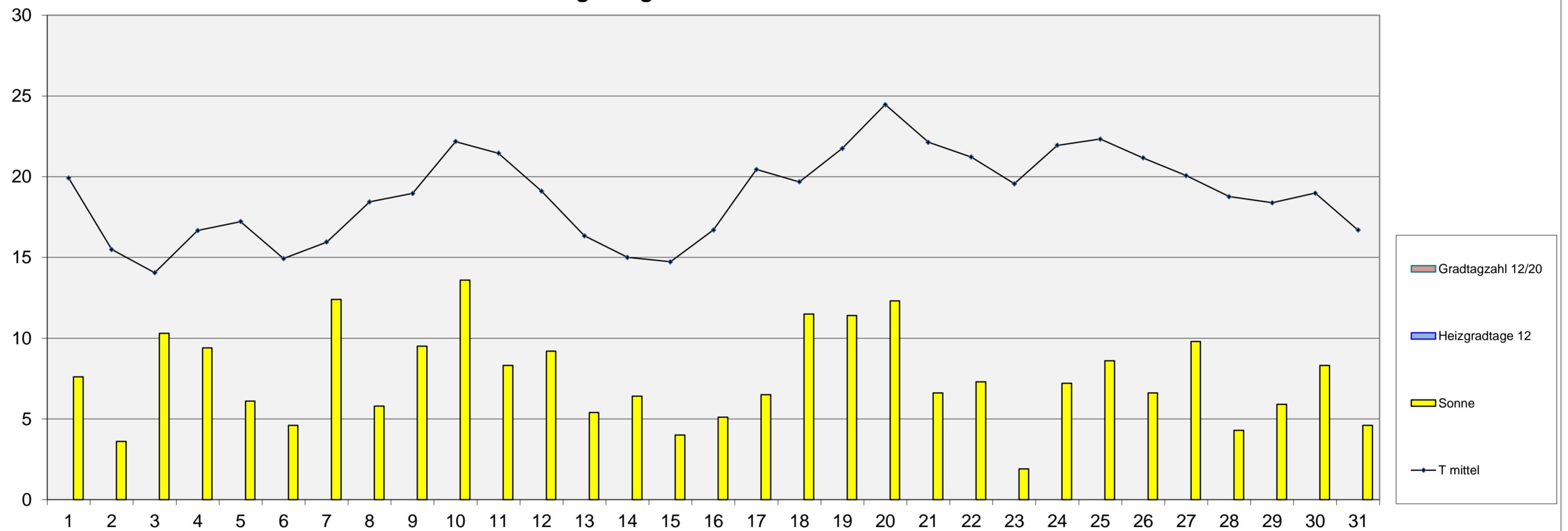
Energiediagramm Juli 2016
